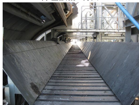
水平コンベヤ テール部
